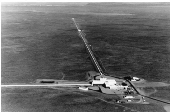
LIGO 项目的巨型装置，目的只是为了探测引力波
