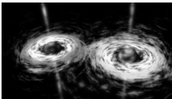
十三亿光年外,两个黑洞“碰撞”
